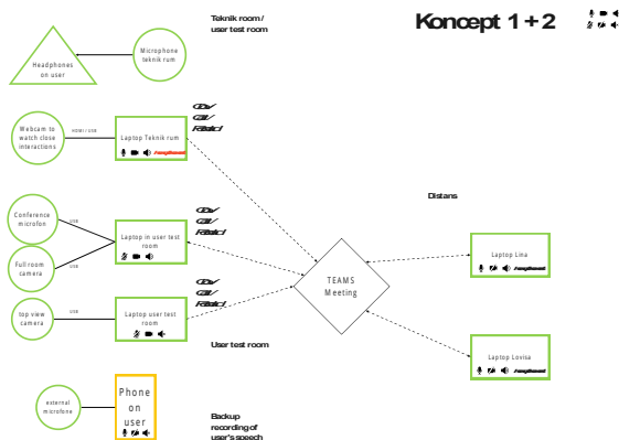
Bild 2. Tekniskt schema
